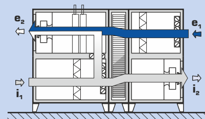
Mod combinat (ventilație cu recirculare)
